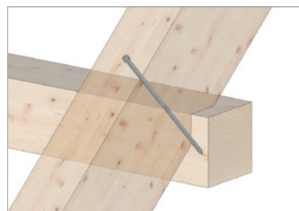
Assemblages chevrons-pannes
